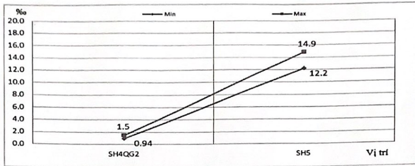
Hình 2: Biểu đồ độ mặn trên sông Hiếu
